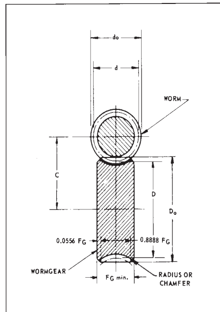
FIGURE 2.6 — WORM & WORMGEAR
