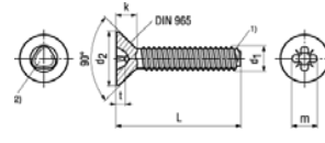
Flat Pozidriv® Type M
