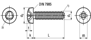
Pan Pozidriv® Type C
