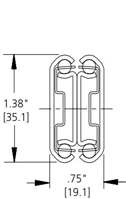
204A-LR 140 lbs./pr. [64 kg]
