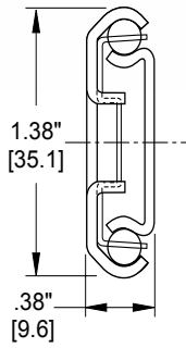
204A-LR 140 lbs./pr. [64 kg]
